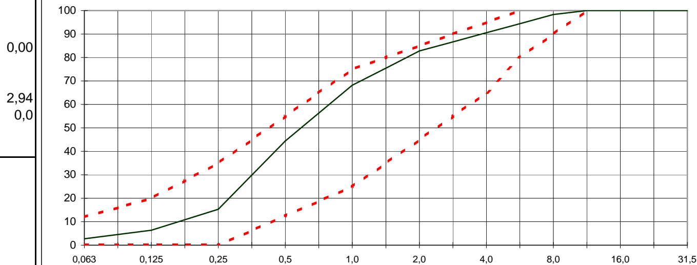
Begränsningslinjer enl. SS 13 21 01
