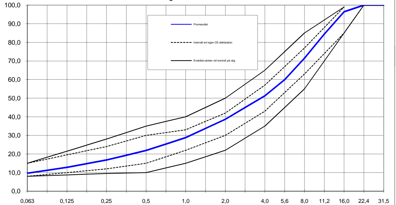
Grusslitlager enl VVTBT 2007:117
