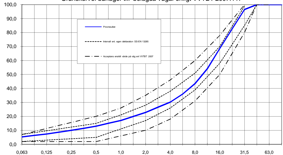
Gränskurvor bärlager till belagda vägar enligt VVTBT 2007:117
